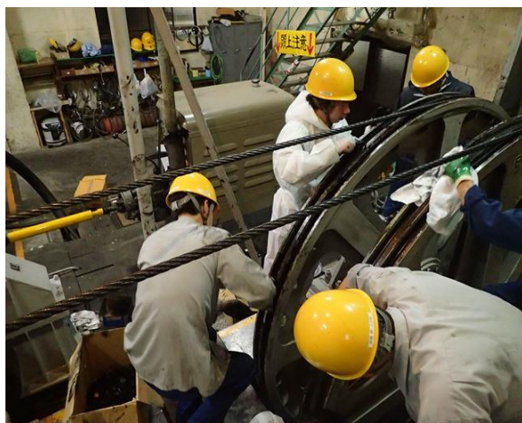
対動滑車ゴムブロックライナー交換作業
