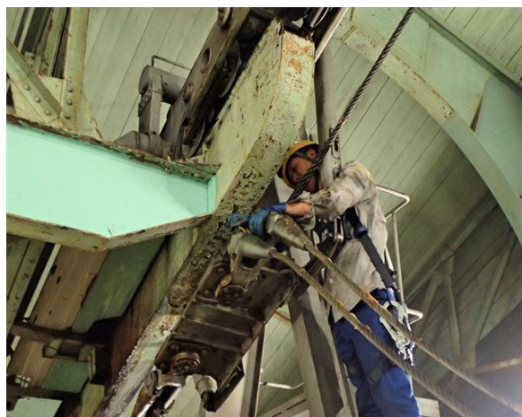
曳索切り詰め作業（山頂駅）
